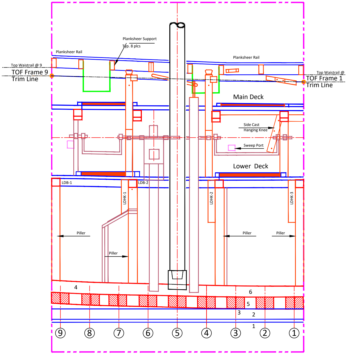
Longitudinal Section 1:48
